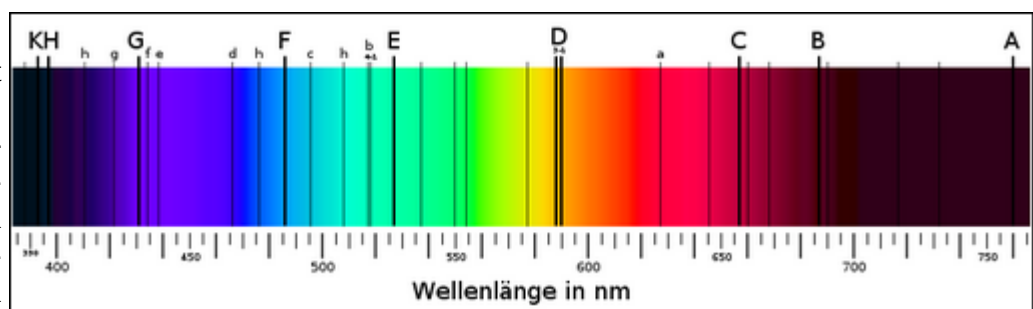
Die wichtigsten Fraunhoferlinien im sichtbaren Bereich des elektromagnetischen Spektrums. [Nach wikipedia.org .]
