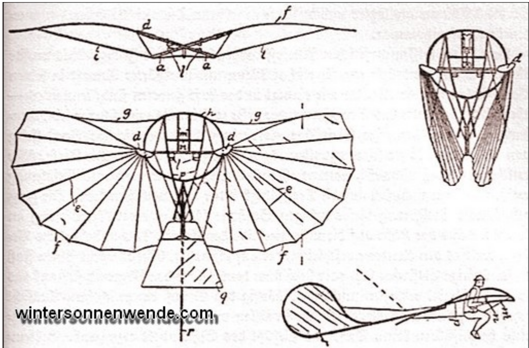
[285] Konstruktionszeichnungen Otto Lilienthals für ein Gleitflugzeug. Aus seiner Patentschrift vom 1. September 1893.
