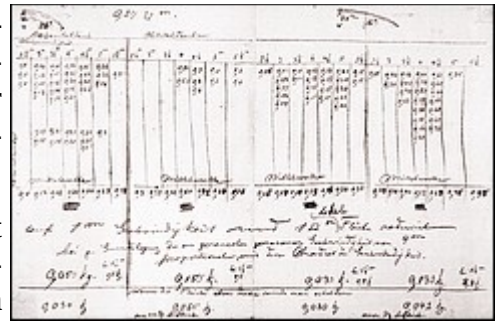
Lilienthals Auftriebsmessungen an gewölbten Flächen mit Anstellwinkeln von 26 und 16 Grad mit Vergleich zu offensichtlich vorher ermittelten Werten an ebenen Flächen.
