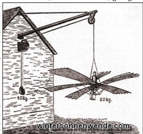
[277] Von den Brüdern Lilienthal 1867 konstruierter Schlagflügelapparat , mit dessen Hilfe sie die Hebewirkung von Flugzeugflügeln feststellten. Aus Otto Lilienthals Buch "Der Vogelflug als Grundlage der Fliegekunst", 1889.
