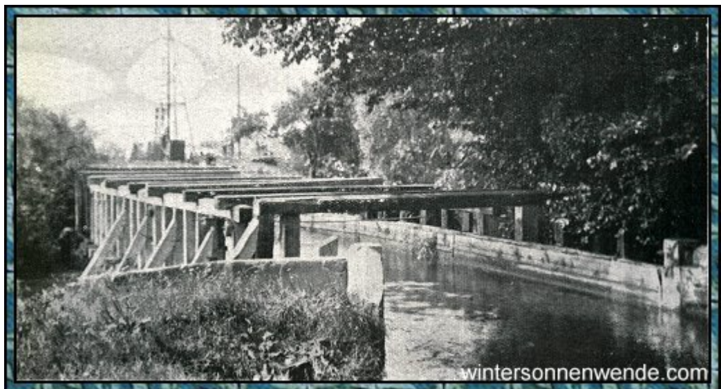
Die Riedwand bei Herrengrebin. Blick von oben auf die übergeleitete Kladau. Ergänzung zum vorhergehenden Bild. Entnommen mit Genehmigung des Deichverbandes: Bertram - La Baume - Kloeppe, "Das Weichsel-Nogat-Delta."
